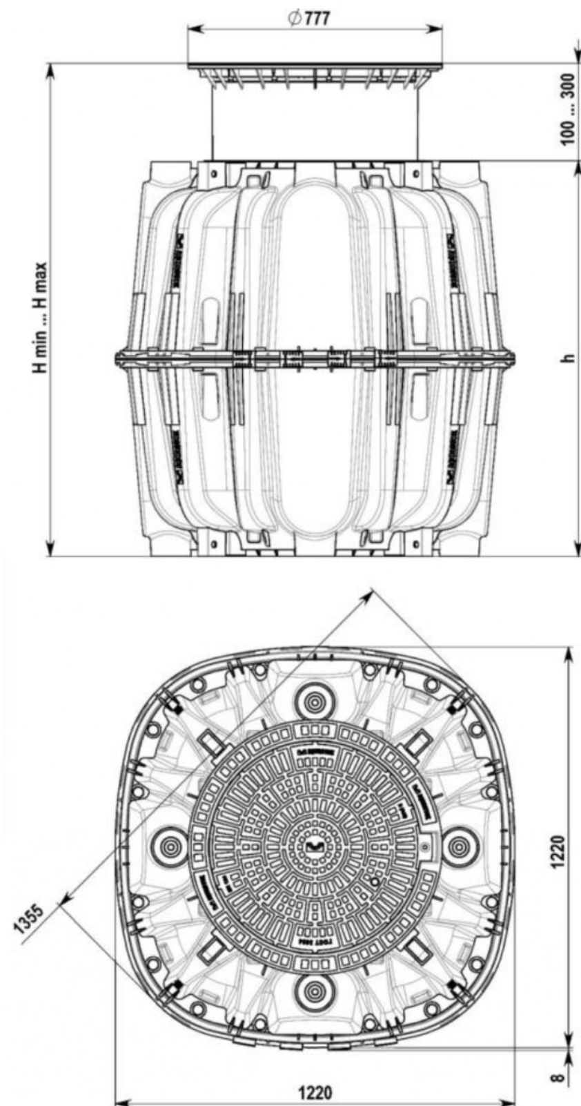
Рисунок 2 – Основные геометрические характеристики полимерного колодца универсального.
