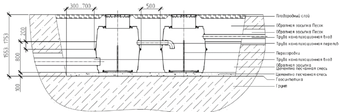
Рисунок 8 – системы отстойника и очистки ливневых и канализации.
