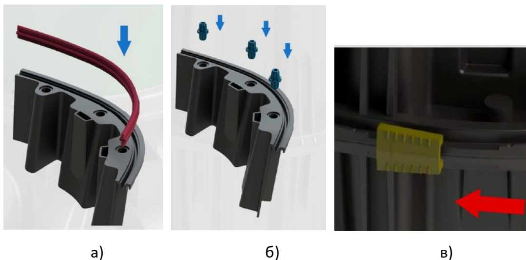
Рисунок 11 – Этапы сборки колодца
