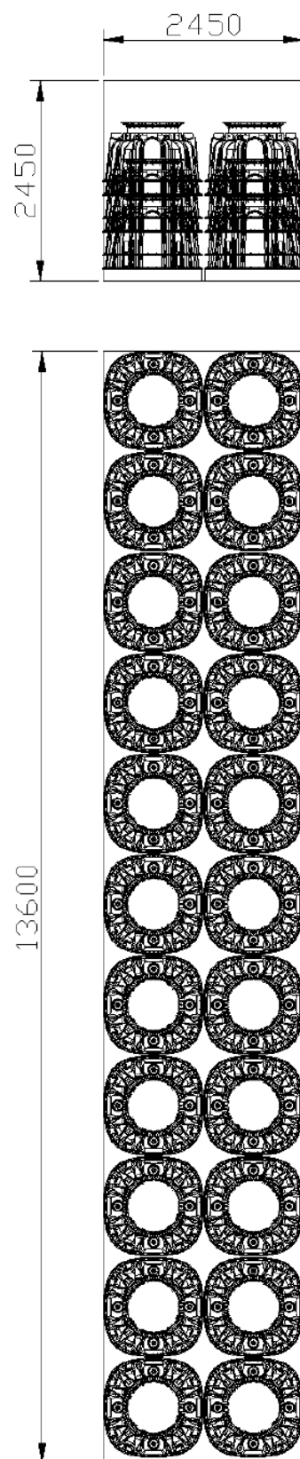
Рисунок 13 – Размещение колодцев в полуприцепе. 11 рядов х 6 комплектов в ряду = 66 комплектов.
