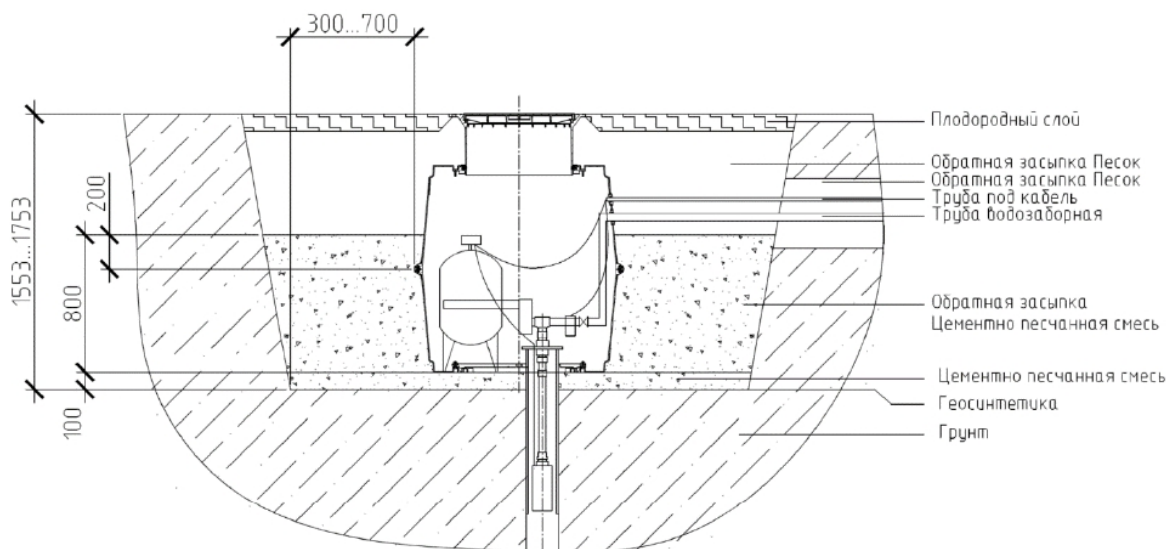
Рисунок 7 – Смотровой колодец с оборудованной скважиной.
