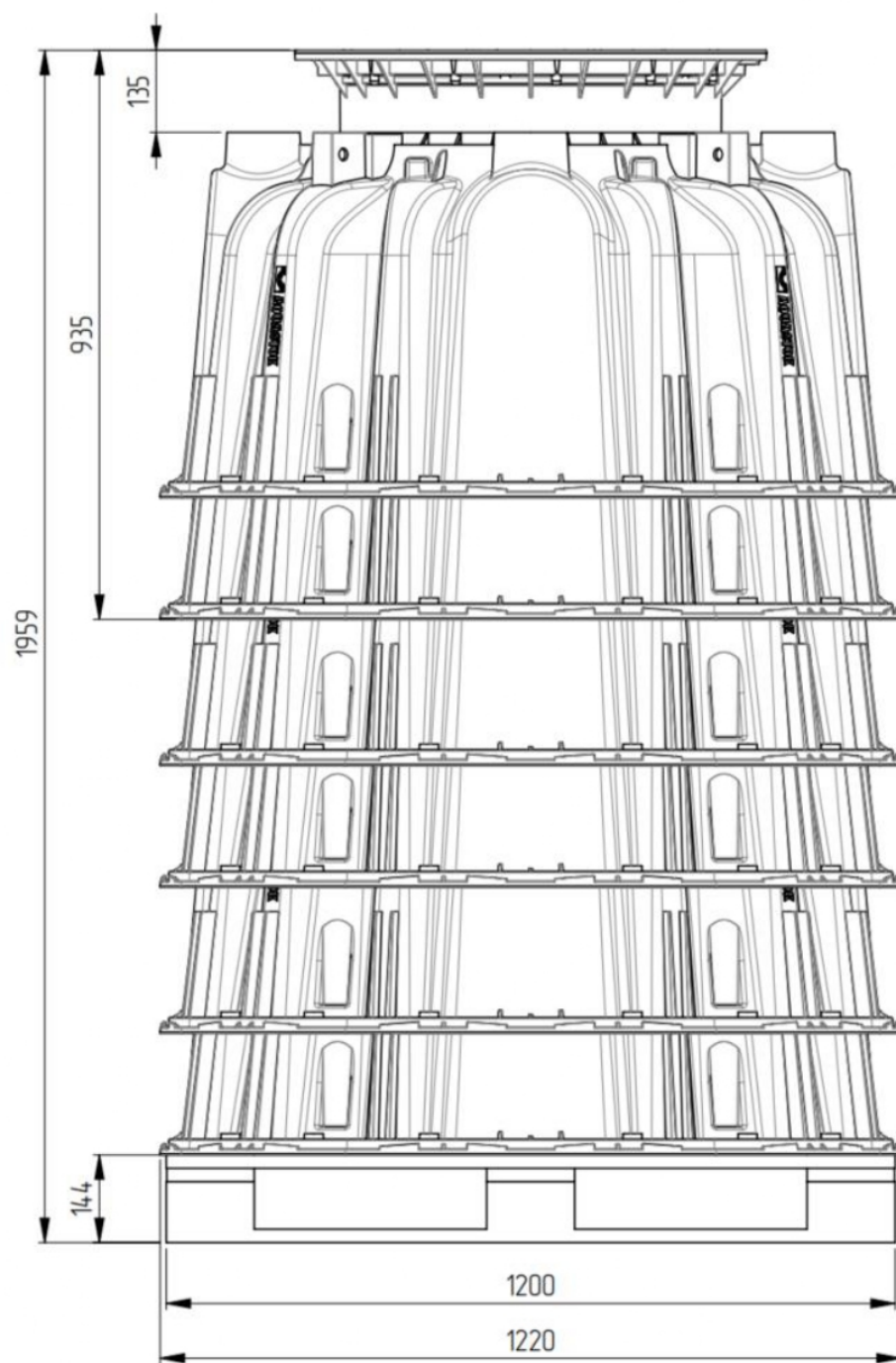
Рисунок 12 – Укладка трех комплектов на поддоне
