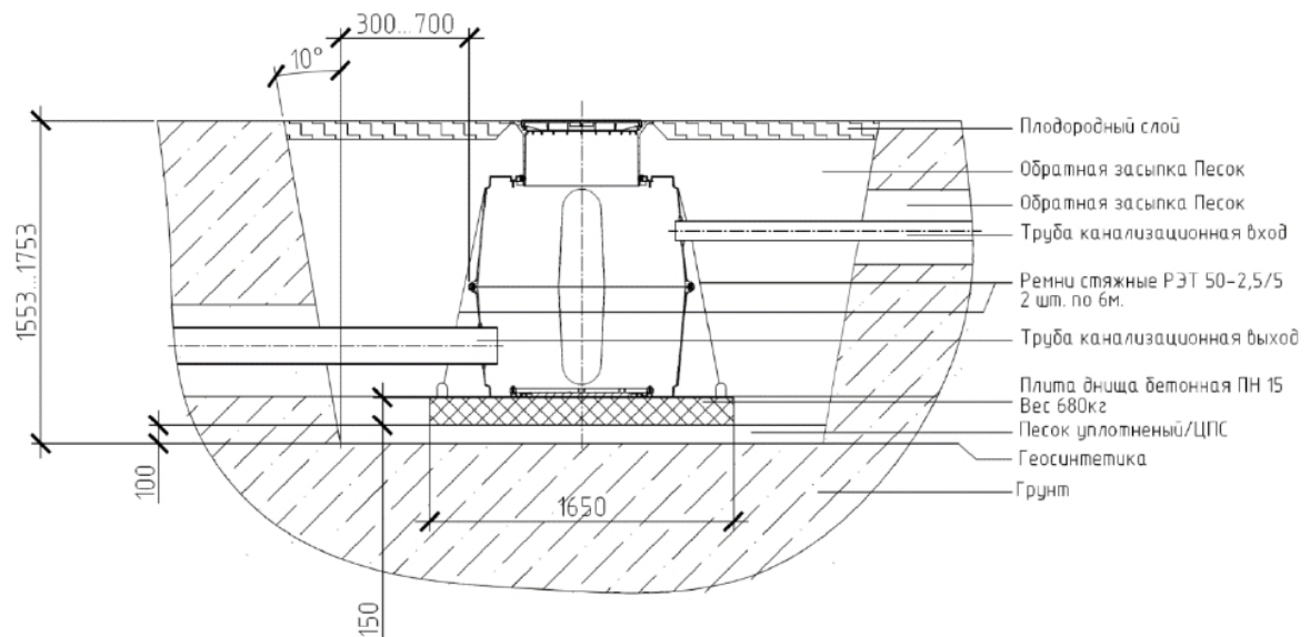
Рисунок 4 – Канализационный колодец на железобетонной плите.
