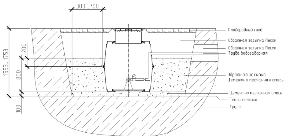
Рисунок 6 – Смотровой колодец с приборами учета водоснабжения.
